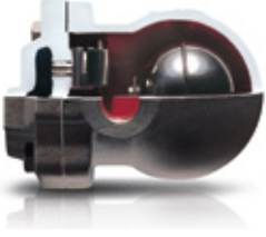
ŞAMANDIRALI KONDENSTOP
