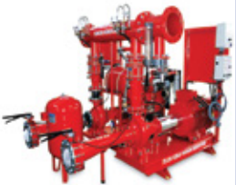
YANGIN HİDROFORU
